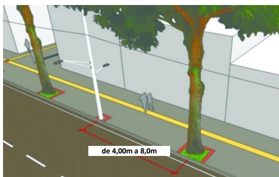
Imagem 2: Distância mínima aos postes da rede aérea.
